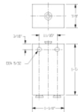
USV-100 Dimensions
