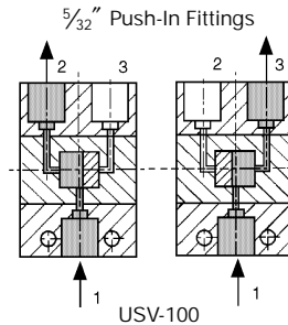
USV-100
